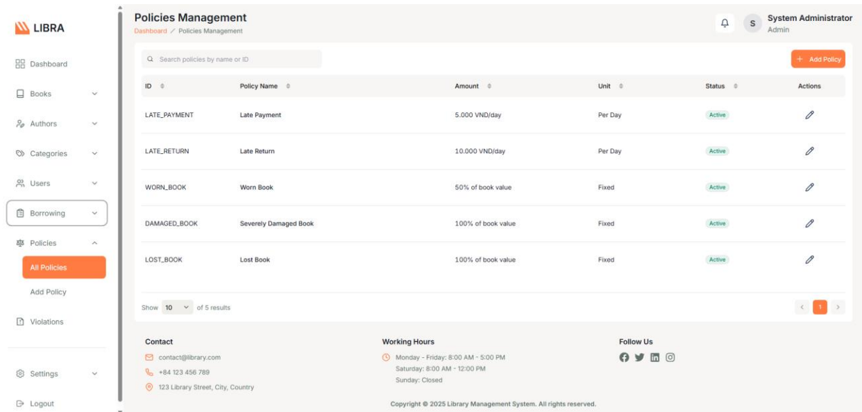
Hình 3.12. Giao diện Quản lý chính sách
