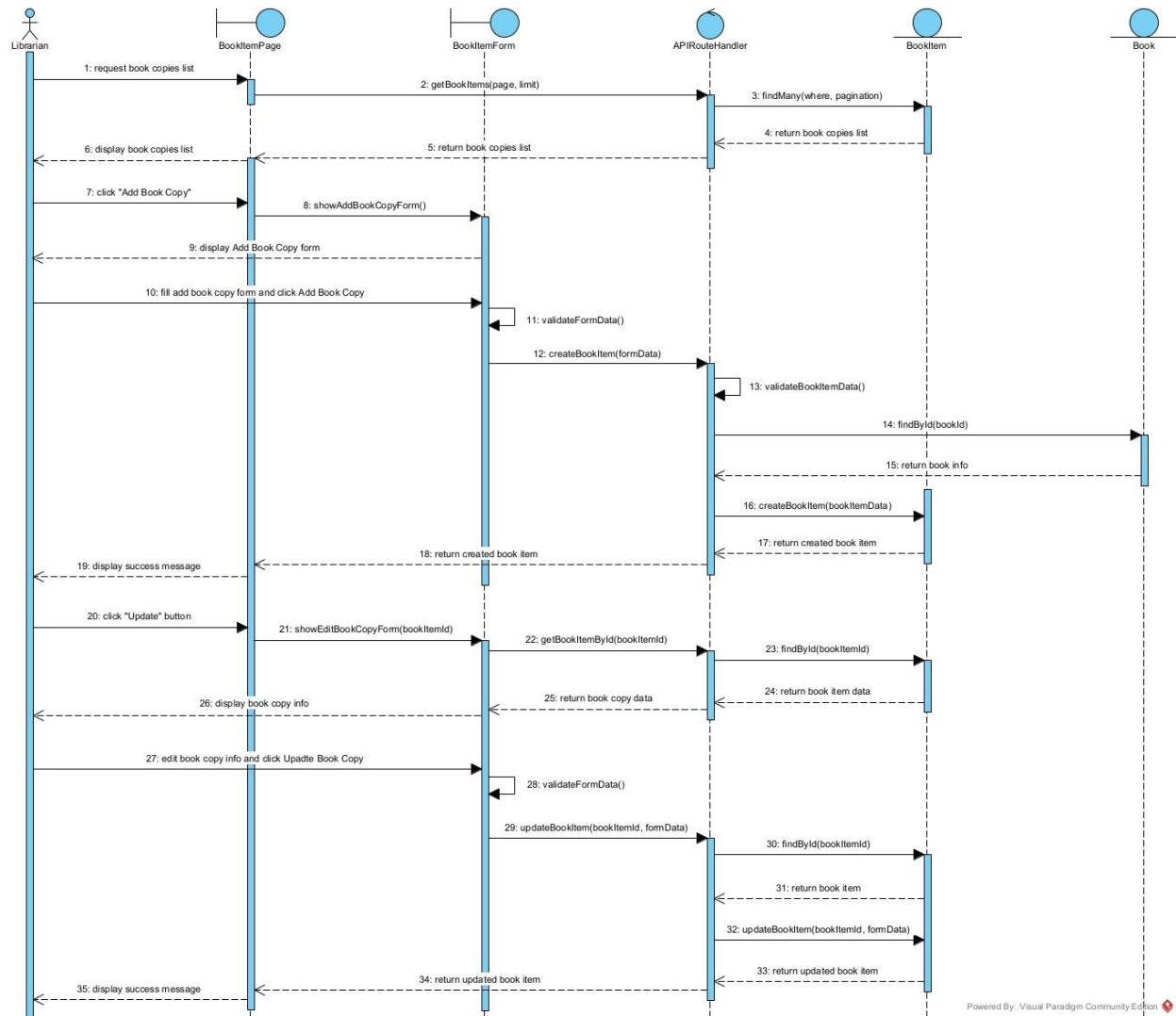
Hình 2.17. Biểu đồ tuần tự cho chức năng Quản lý bản sao sách
