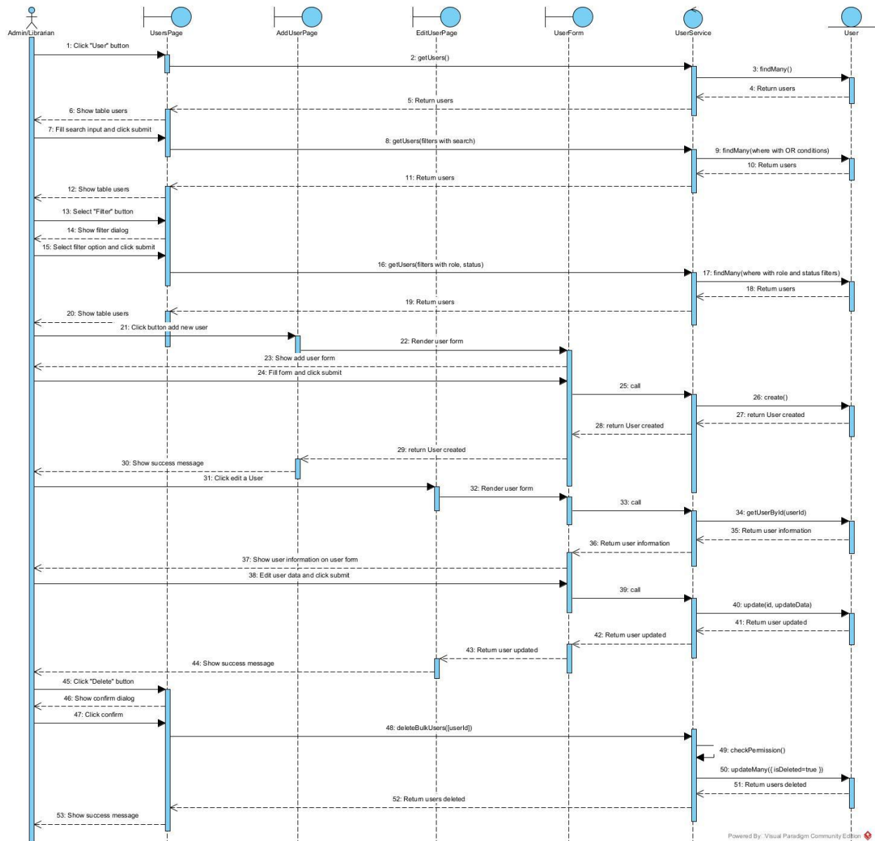
Hình 2.26. Biểu đồ tuần tự cho chức năng Quản lý người dùng
