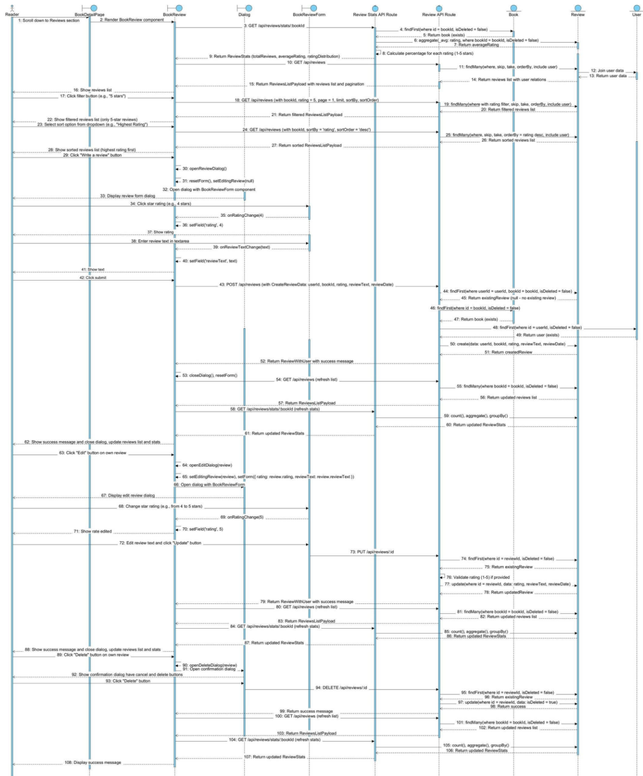
Hình 2.29. Biểu đồ tuần tự cho chức năng Đánh giá sách
