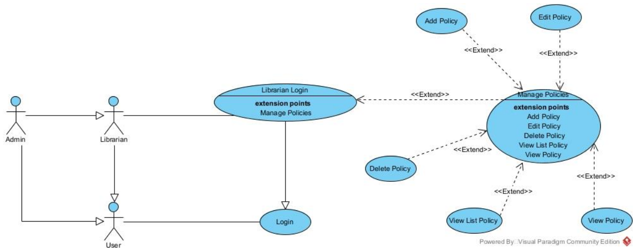
Hình 2.7. Biểu đồ use case chức năng Quản lý chính sách
