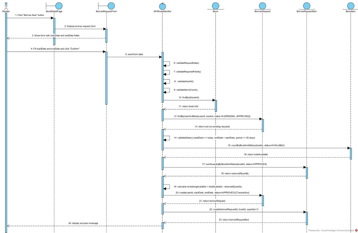
Hình 2.21. Biểu đồ tuần tự cho chức năng Tạo yêu cầu mượn sách
