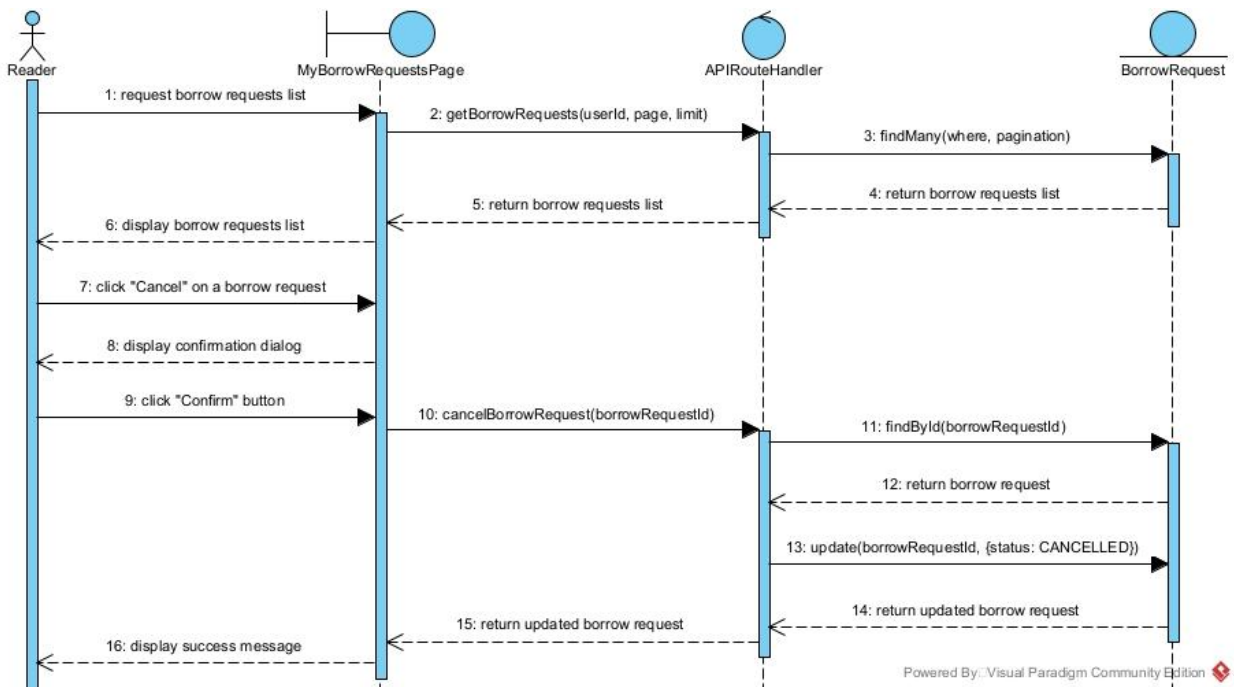
Hình 2.22. Biểu đồ tuần tự cho chức năng Quản lý yêu cầu mượn sách
