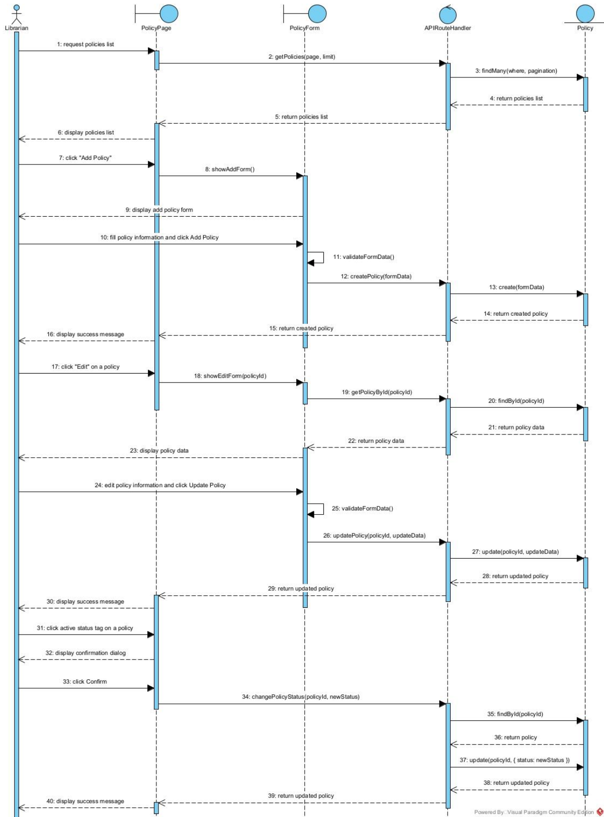
Hình 2.30. Biểu đồ tuần tự cho chức năng Quản lý chính sách
