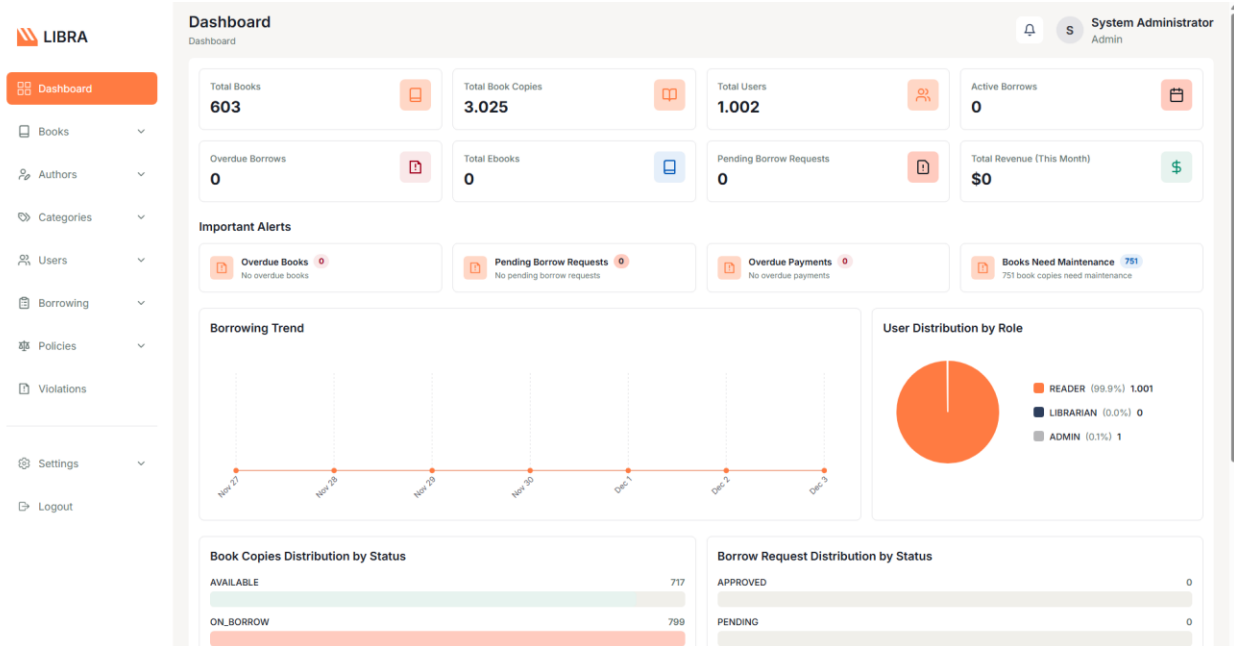
Hình 3.10. Giao diện Thống kê hệ thống
