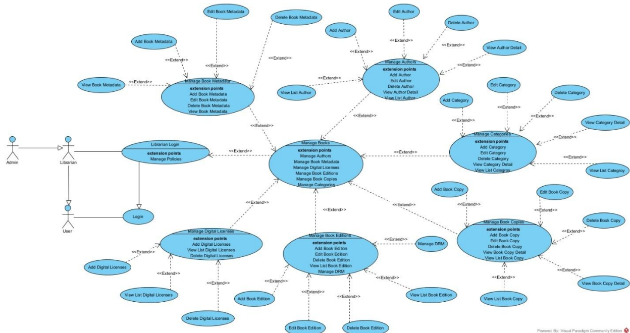
Hình 2.5. Biểu đồ use case chức năng Quản lý sách
