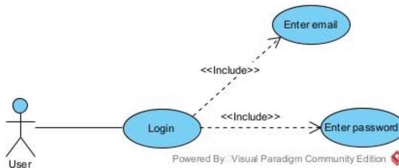
Hình 2.3. Biểu đồ use case chức năng Đăng nhập
