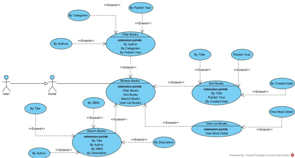
Hình 2.9. Biểu đồ use case chức năng Duyệt sách
