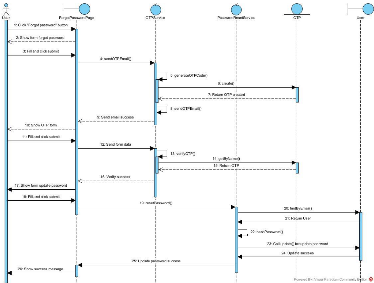
Hình 2.14. Biểu đồ tuần tự cho chức năng Đặt lại mật khẩu
