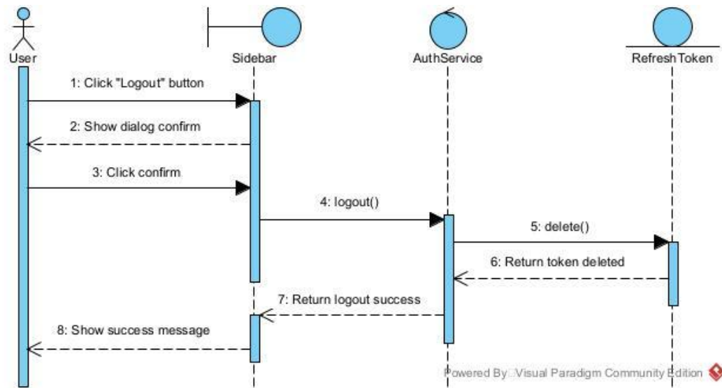
Hình 2.13. Biểu đồ tuần tự cho chức năng Đăng xuất
