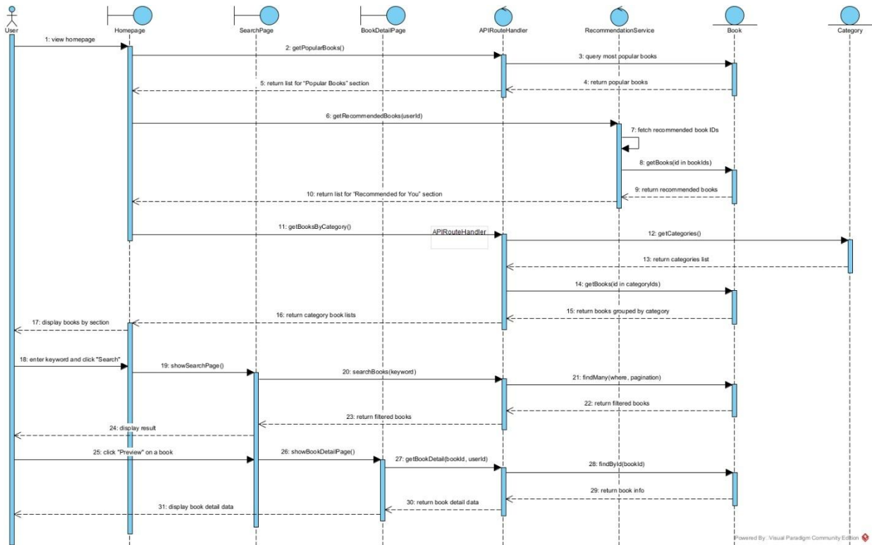
Hình 2.27. Biểu đồ tuần tự cho chức năng Duyệt sách
