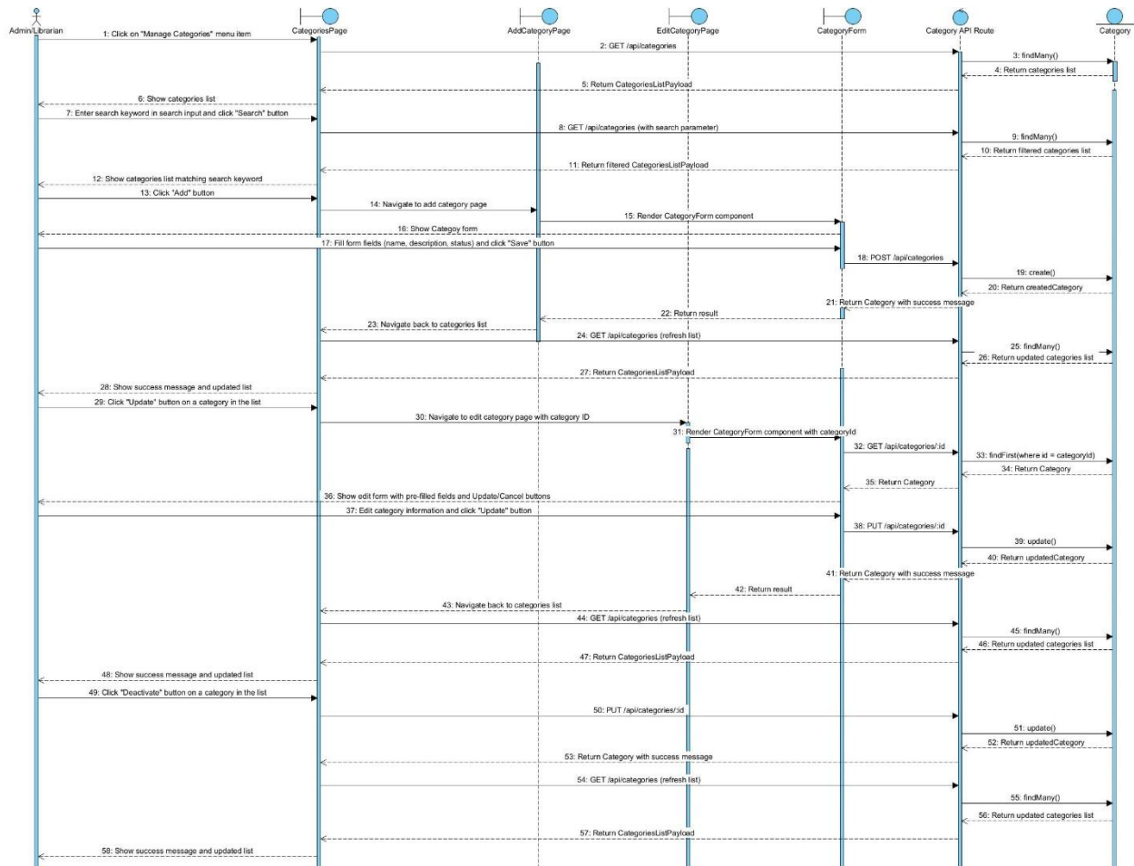
Hình 2.20. Biểu đồ tuần tự cho chức năng Quản lý thể loại sách
