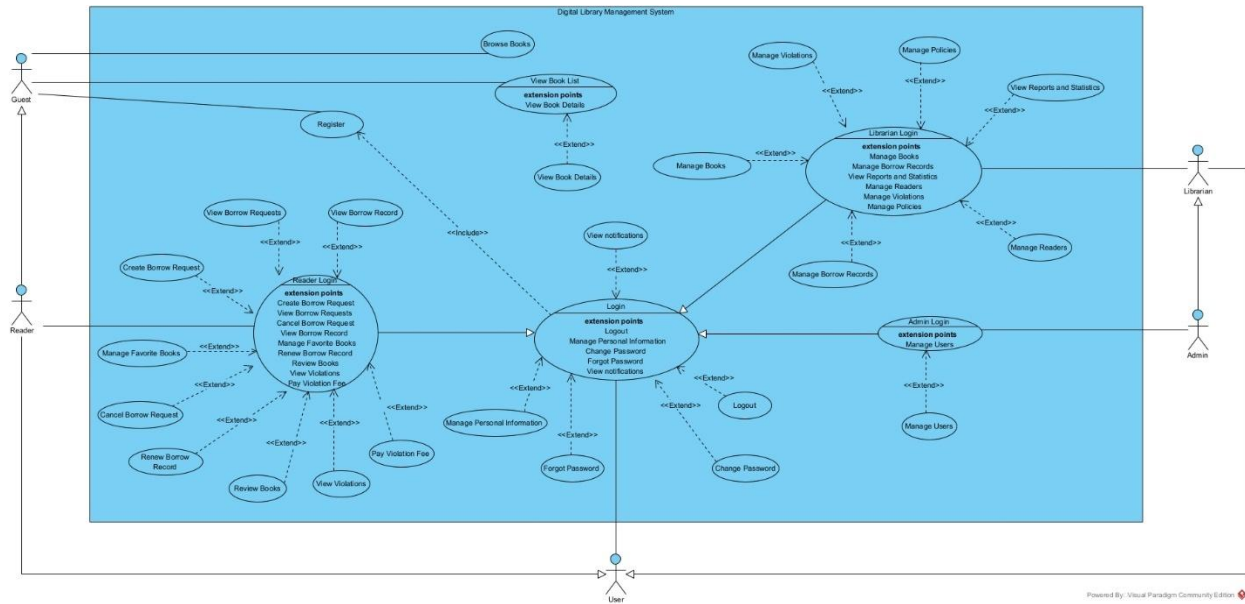
Hình 2.1. Biểu đồ use case tổng quan hệ thống
