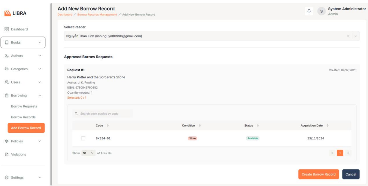
Hình 3.5. Giao diện Tạo phiếu mượn của thủ thư
