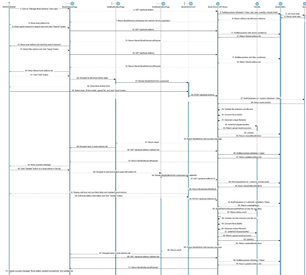
Hình 2.18. Biểu đồ tuần tự cho chức năng Quản lý sách điện tử
