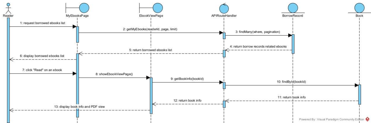
Hình 2.25. Biểu đồ tuần tự cho chức năng Đọc sách điện tử
