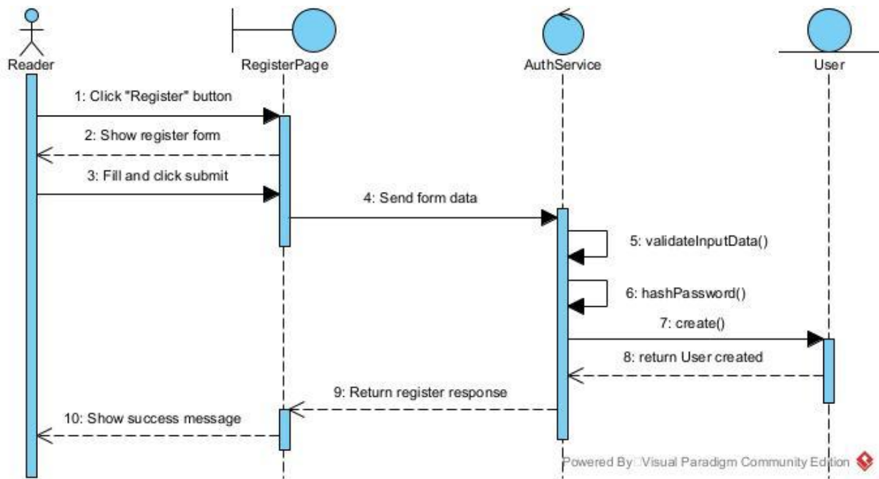
Hình 2.11. Biểu đồ tuần tự cho chức năng Đăng ký
