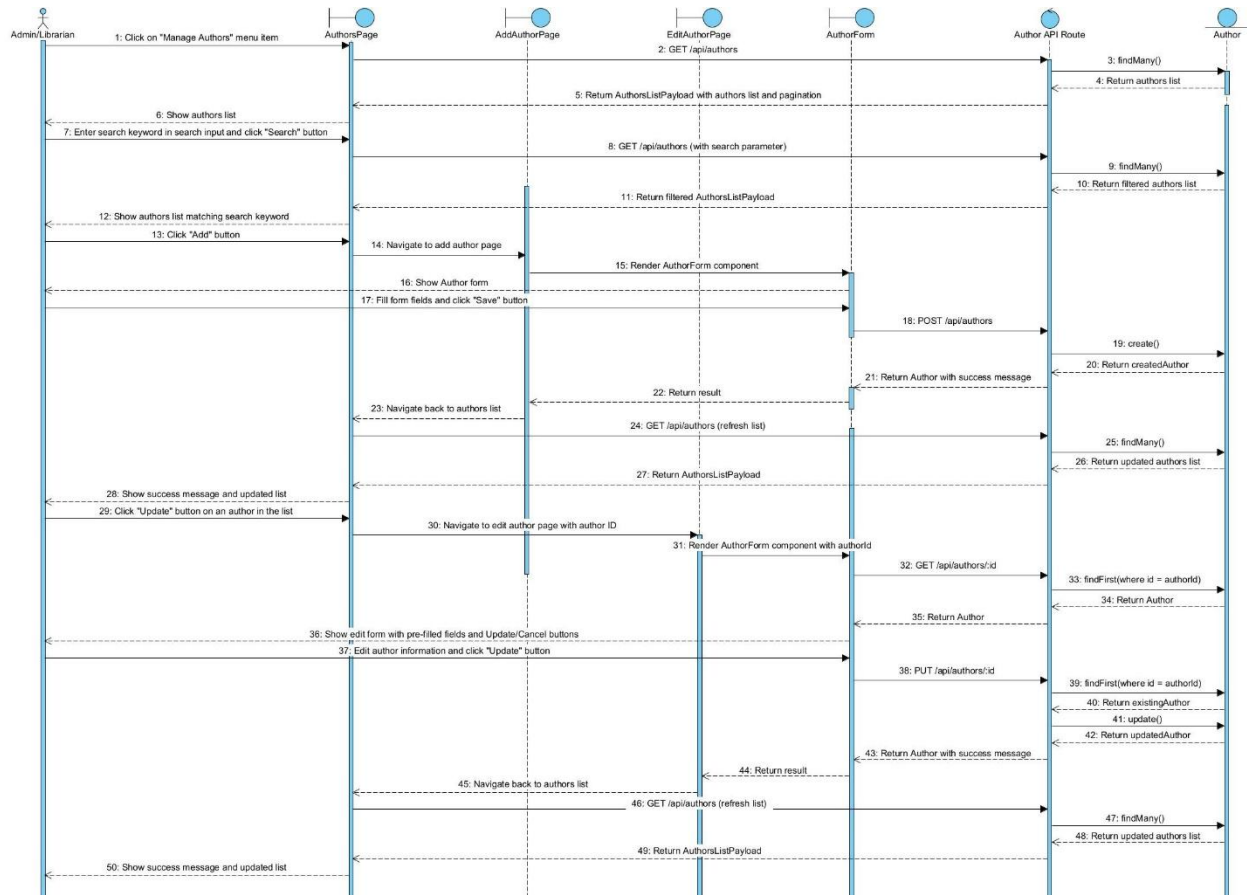
Hình 2.19. Biểu đồ tuần tự cho chức năng Quản lý thông tin tác giả
