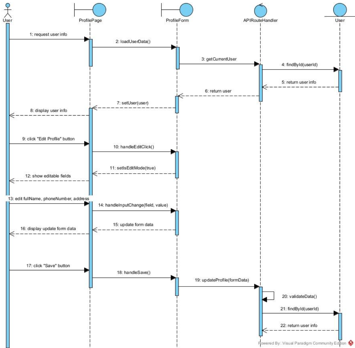
Hình 2.15. Biểu đồ tuần tự cho chức năng Quản lý thông tin cá nhân
