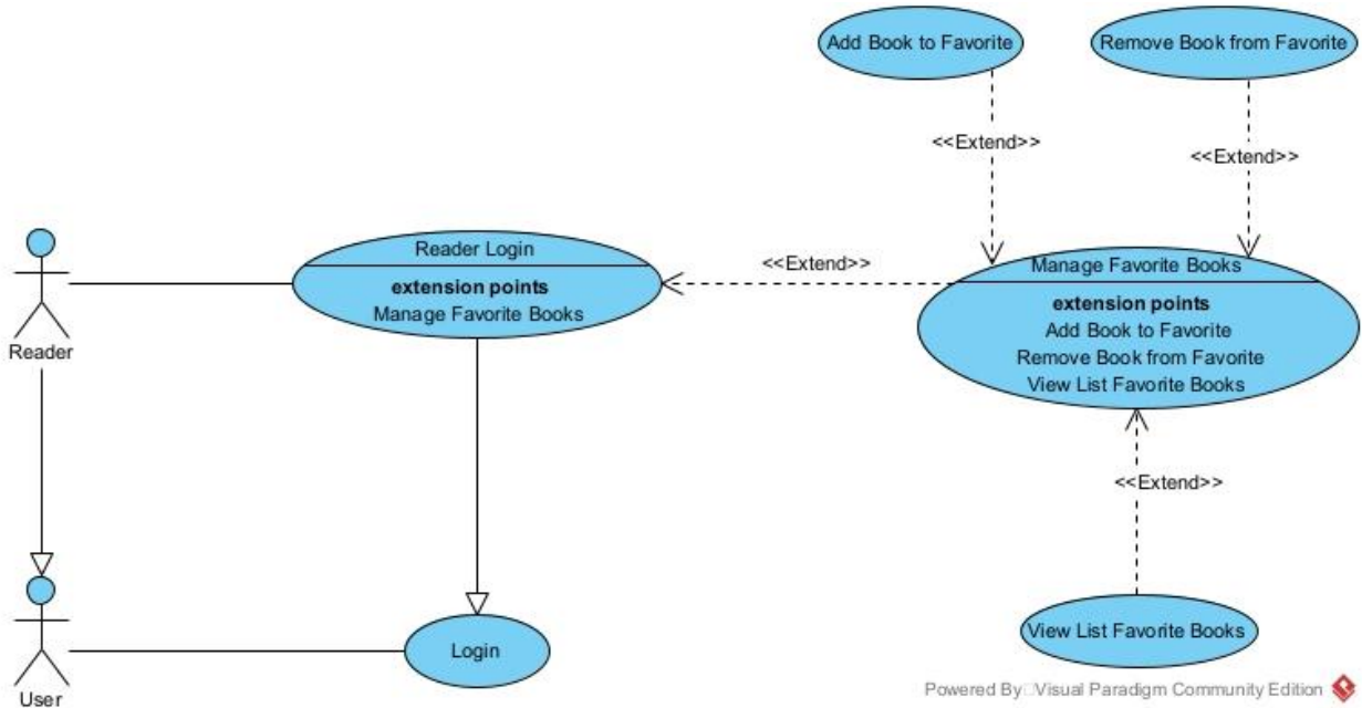
Hình 2.8. Biểu đồ use case chức năng Quản lý sách yêu thích
