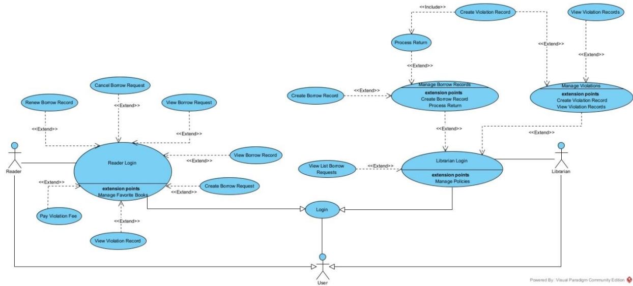
Hình 2.6. Biểu đồ use case Quản lý mượn - trả
