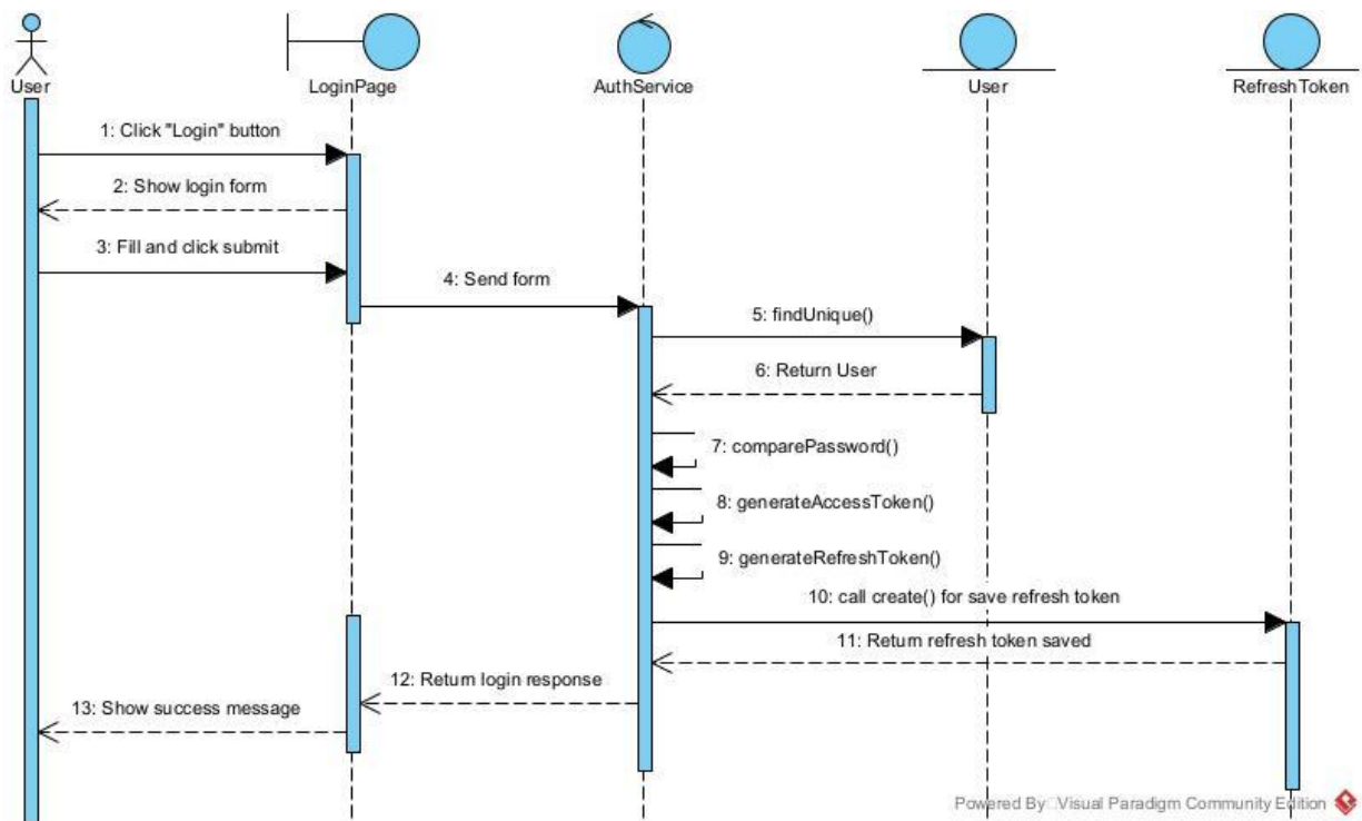
Hình 2.12. Biểu đồ tuần tự cho chức năng Đăng nhập
