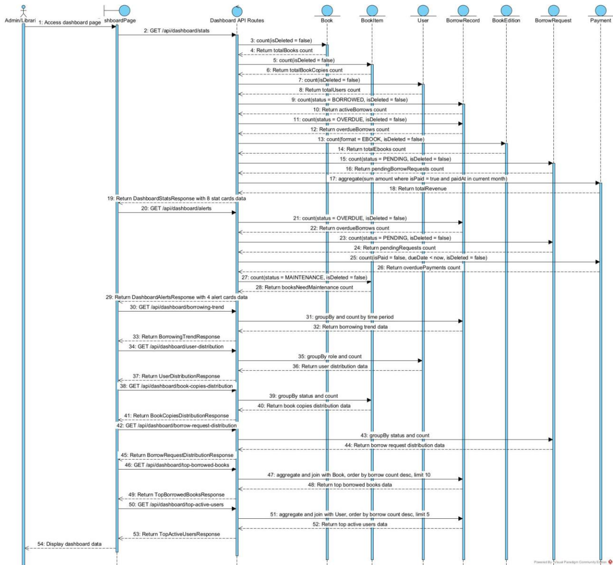
Hình 2.31. Biểu đồ tuần tự cho chức năng Xem thống kê hệ thống
